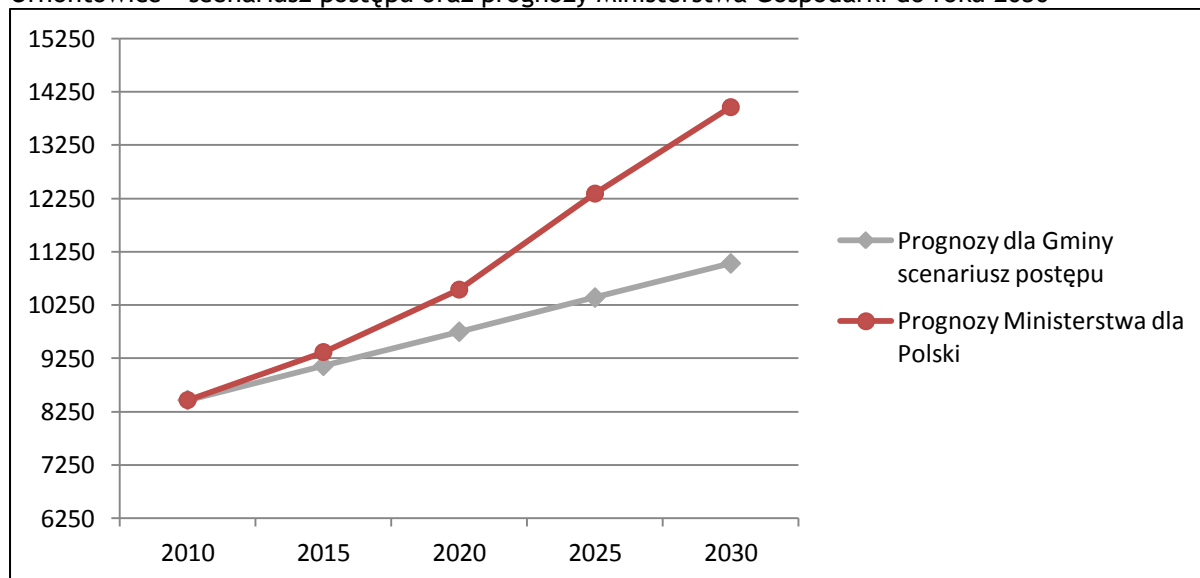
Rysunek 11 Porównanie prognoz zapotrzebowania na energię elektryczną w MWh w przypadku Gminy Ornontowice - scenariusz postępu oraz prognozy Ministerstwa Gospodarki do roku 2030
