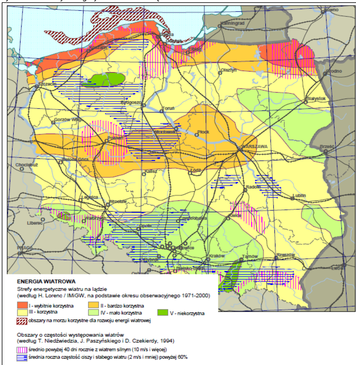
Rysunek 16 Strefy energetyczne wiatru na łądzie
